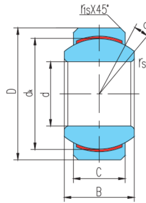
外形尺寸mm
