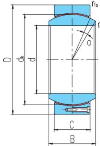
外形尺寸mm
