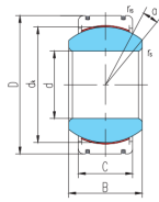
GEG...XT-2RS
